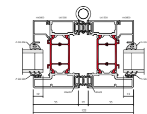
F82 Interlock
