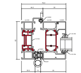
F82 Jamb
