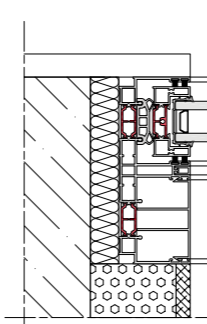
Jamb Detail
