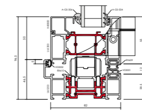
F82 Cill
